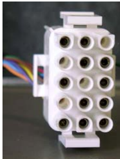
15 pins AMP-f 24 Volt (EUR-941)
